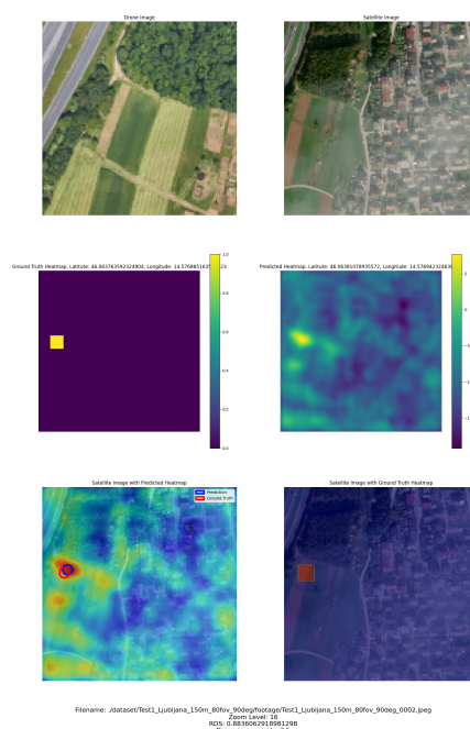
Slika 4.5: Primer izhoda ob uporabi Hanningove kriterijske funkcije
