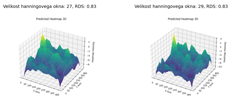
Slika 4.13: Primerjava toplotnih map ob uporabi velikosti 27 in 29 Hanningovega okna.
