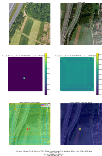
Slika 4.7: Primer izhoda ob uporabi Hanningove utežene srednje kvadratne napake
