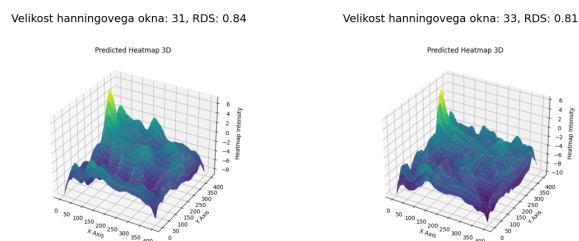
Slika 4.12: Primerjava toplotnih map ob uporabi različnih velikosti Hanningovega okna.
