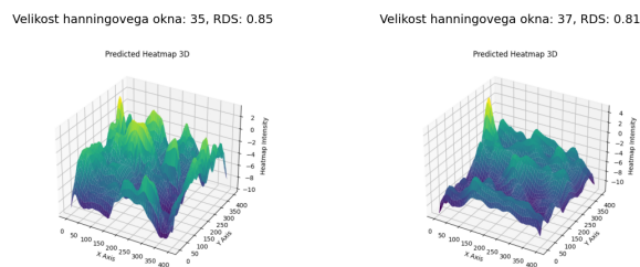
Slika 4.13: Primerjava toplotnih map ob uporabi različnih velikosti Hanningovega okna.
