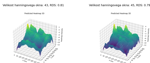
Slika 4.15: Primerjava toplotnih map ob uporabi različnih velikosti Hanningovega okna.
