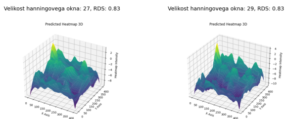
Slika 4.11: Primerjava toplotnih map ob uporabi različnih velikosti Hanningovega okna.
