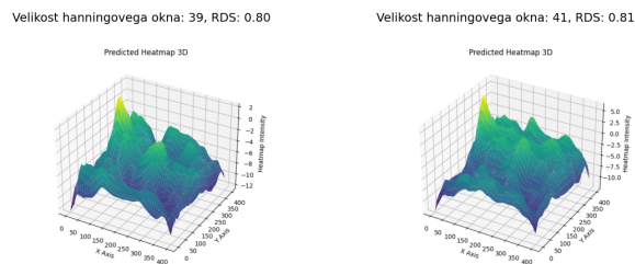
Slika 4.14: Primerjava toplotnih map ob uporabi različnih velikosti Hanningovega okna.
