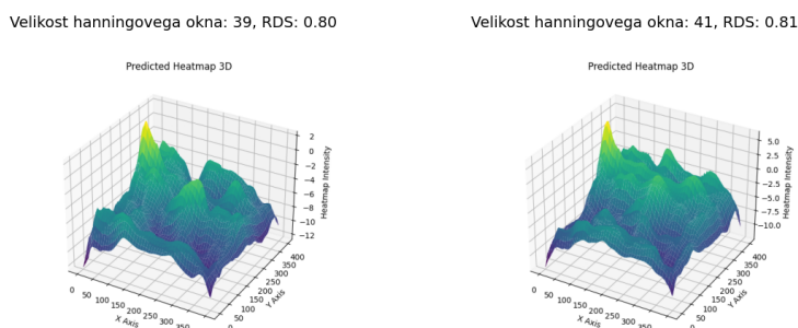
Slika 4.16: Primerjava toplotnih map ob uporabi velikosti 39 in 41 Hanningovega okna.
