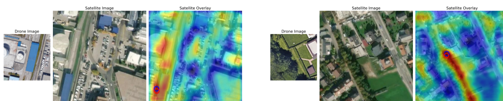
Slika 4.6: Leva slika prikazuje izsek avtoceste z napako 6.55m in RDS vrednostjo 0.91. Desna slika okolico stanovanjske hiše v naselju z napako 5.73m in RDS vrednostjo 0.90.
